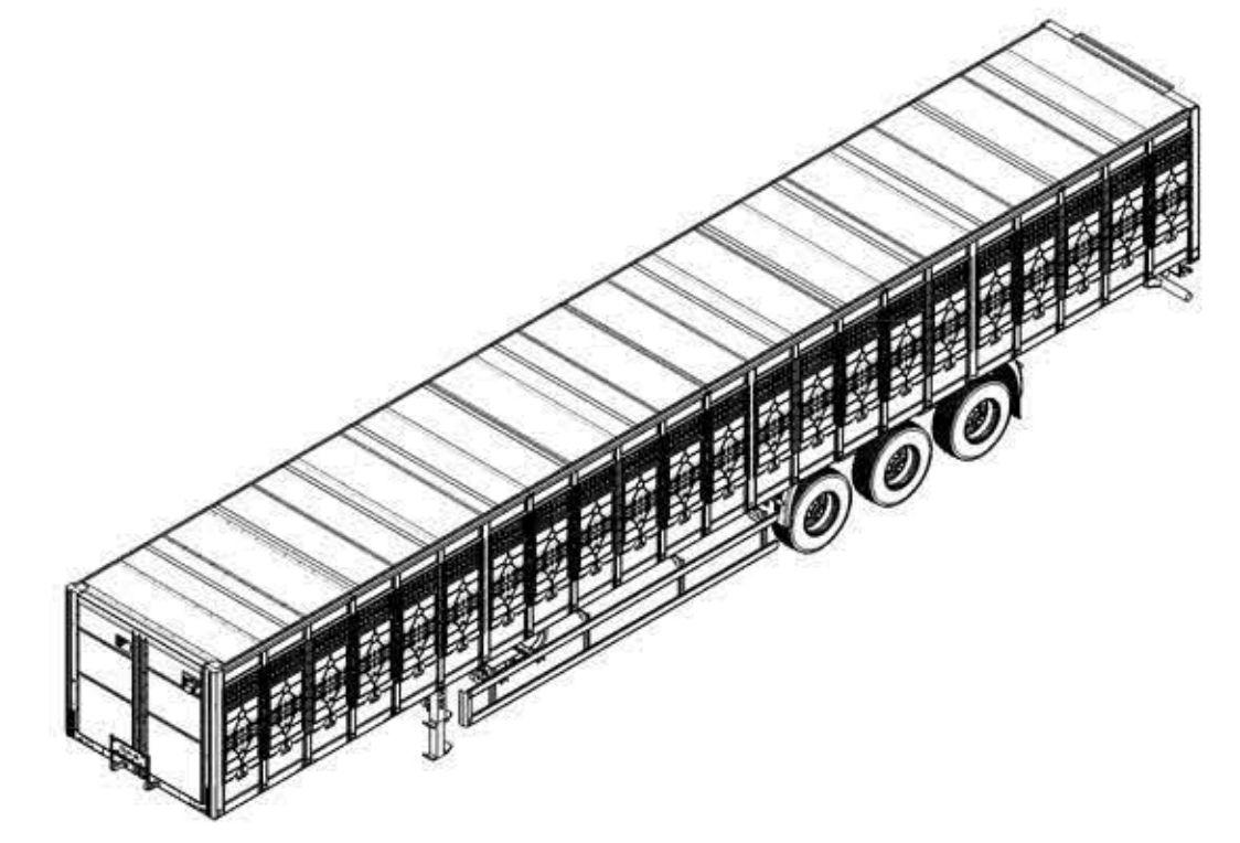
Изометрия (1:100)
